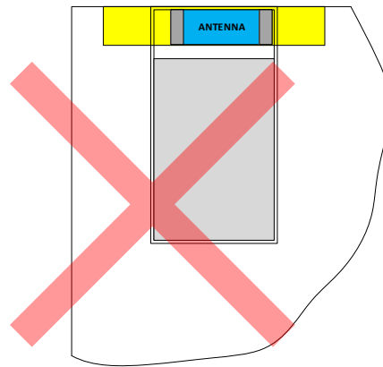
Antenna 영역을 크기를 임의로 조정 또는 Antenna 영역에 GND가 겹치는 형태
