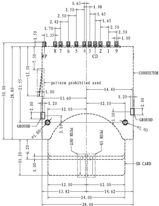
P.C.B LAYOUT
