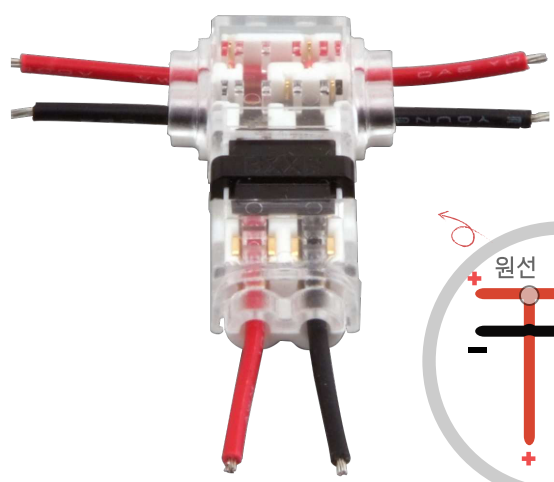
무탈피 2:2 개별분선 T2-2
