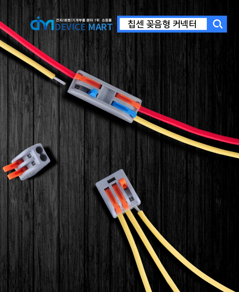
꽃음형커넥터 PCT-2-4
