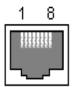
그림 A-1. RJ45 커넥터의 핀 배치
