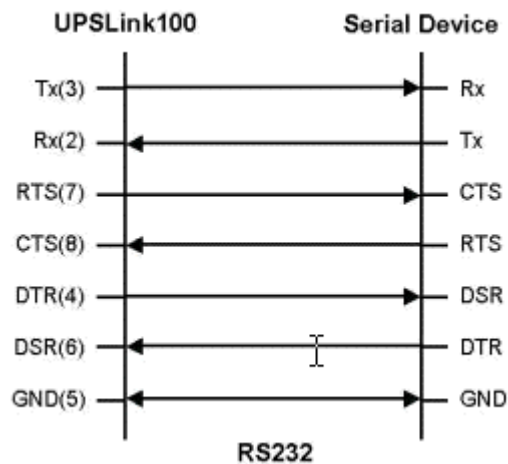
Figure 0-5 RS232 결선도
