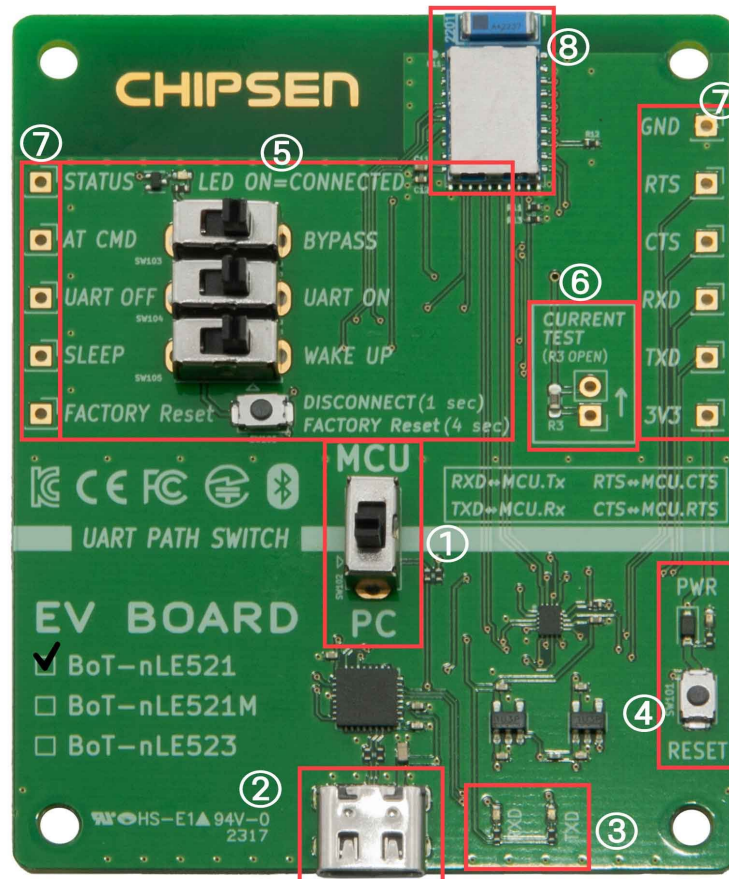
< EVB-nLE521 배치 이미지 >
