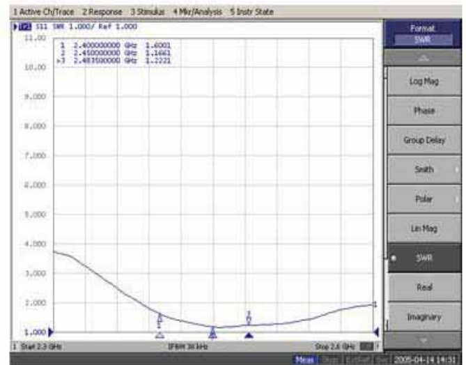
▲ V.S.W.R
