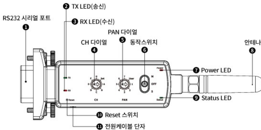
그림 1: RCPort-TD900 외관
