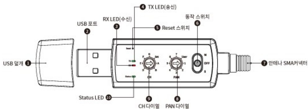
그림 2: RCPort-TD930 외관
