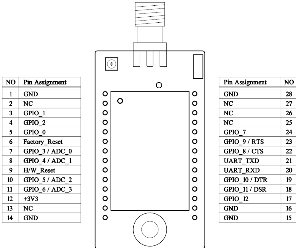
그림 1-2 핀 배치도
