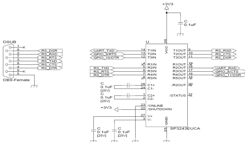
그림 5-3 RS232 시리얼
