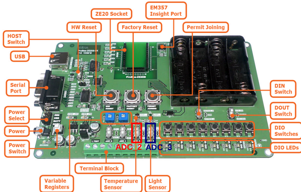
그림 6-6 하드웨어 설정
