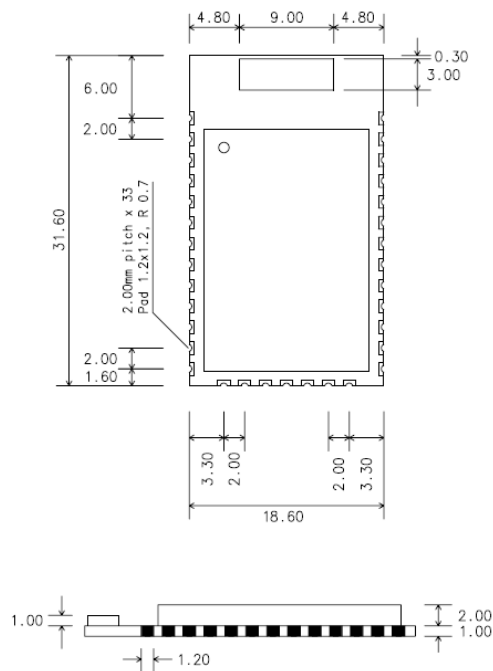
그림 11-5 ProBee-ZE20SSC 치수
