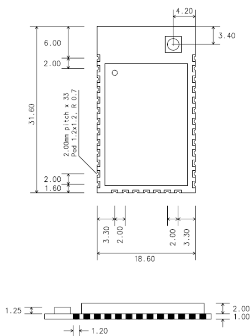
그림 11-4 ProBee-ZE20SSU 치수
