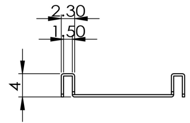
(정면도)
