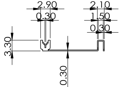
(정면도)
