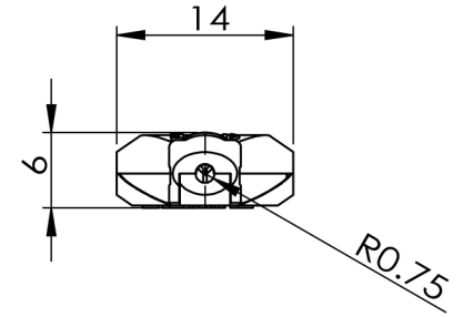
(측면도)
